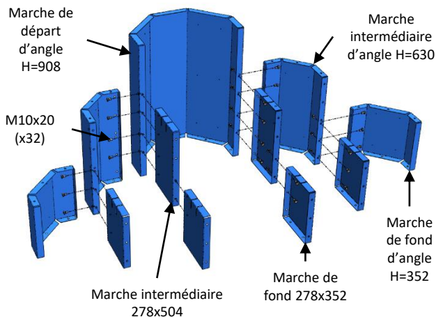
Escalier 3 marches pour piscine hauteur 130
