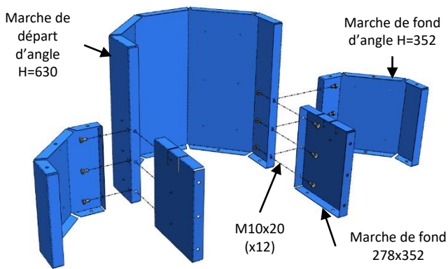
Escalier 2 marches pour piscine hauteur 106
