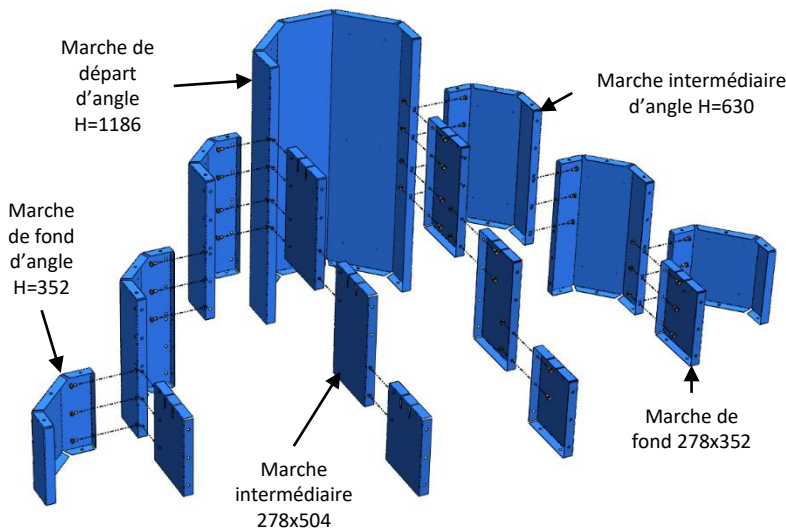
Escalier 4 marches pour piscine hauteur 150
